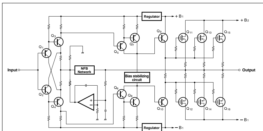
Power MOS-FETs
