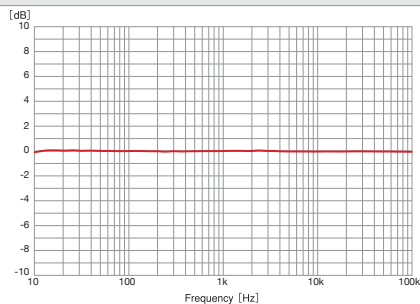
RIAA deviation (MC input)
