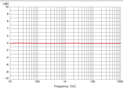
RIAA deviation (MM input)
