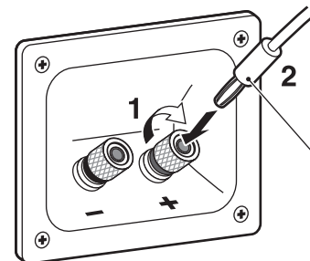
Bananenstecker
