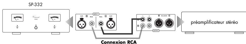
Connexion RCA
