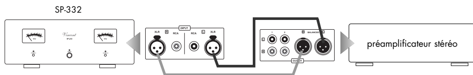
Connexion XLR
