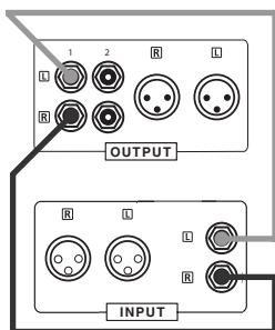
Connexion 1 amplificateur final
