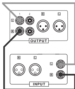
Anschluss 1 Endverstärker
