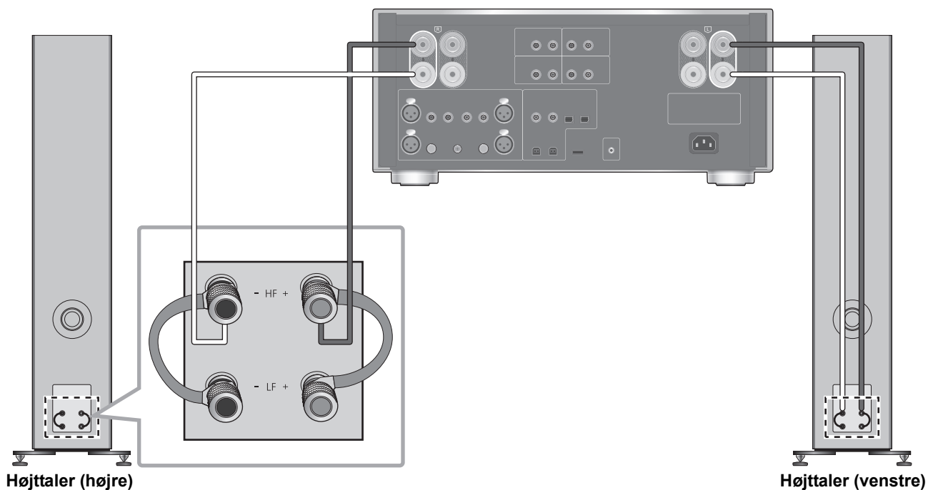
Forstærker (Bag)
