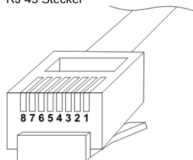
RJ 45 Stecker
