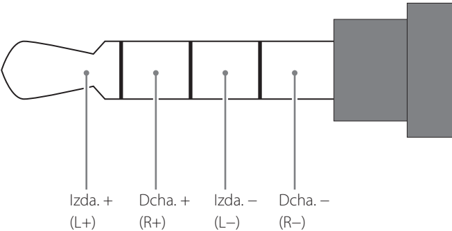
Ilustración del cableado
