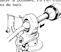
Figure 4. Installing Counter-Weights Abbildung 4. Einbau der Gegengewichte Figure 4. Installation du compteur de poids
