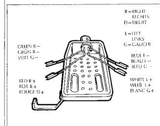
Figure 6. Cartridge Installation Abbildung 6. Einbau der Tonkapsel Figure 6. Installation de la cartouche
