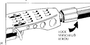
Figure 3. Fitting The Headshell Abbildung 3. Anbringen des Tonkopfes Figure 3. Fixation du manteau de tête
