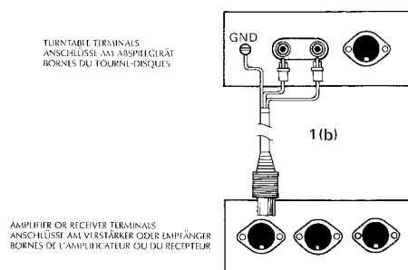
Abbildung 5. Anschließen
