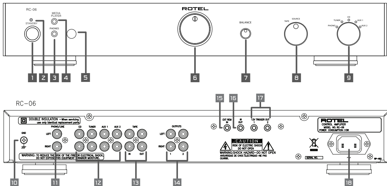
Figure 1: Controls and Connections Commandes et branchements Bedienelemente und Anschlüsse Pannello frontale e posteriore Controles y Conexiones De bedieningsorganen en de aansluitingen Funktioner och anslutningar Органы управления и разъемы
