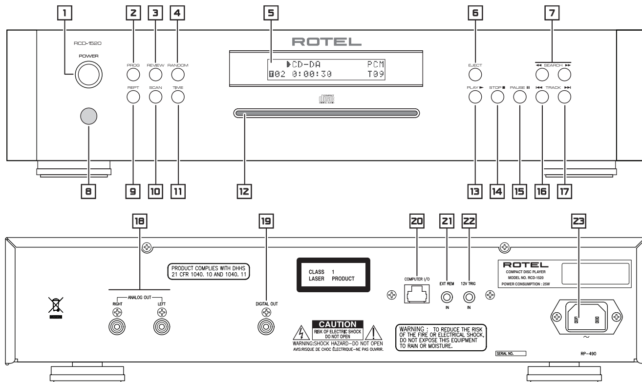
Figure 1: Controls and Connections Commandes et branchements Bedienelemente und Anschlüsse Controles y Conexiones De bedieningsorganen en aansluitingen Controlli e connessioni Funktioner och anslutningar Органы управления и разъемы
