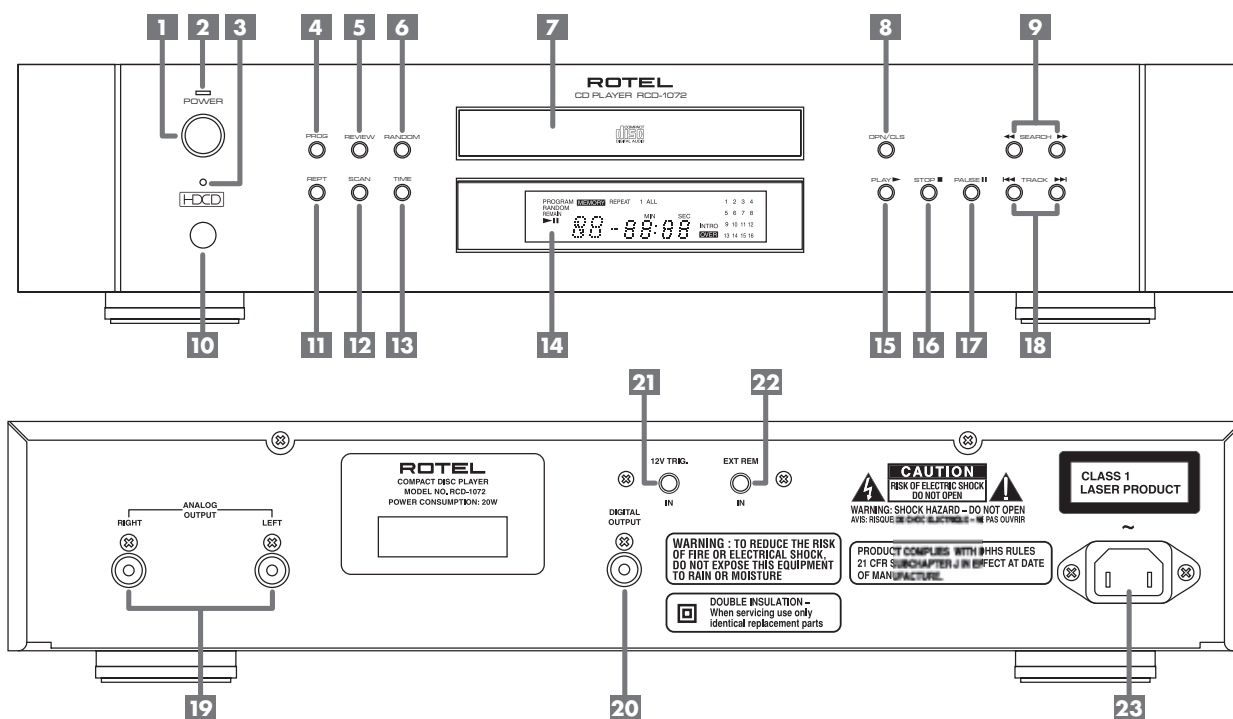
Figure 1: Controls and Connections Commandes et branchements Bedienelemente und Anschlüsse Controlli e collegamenti Controles y Conexiones Bedieningsorganen en aansluitingen Funktioner och anslutningar
