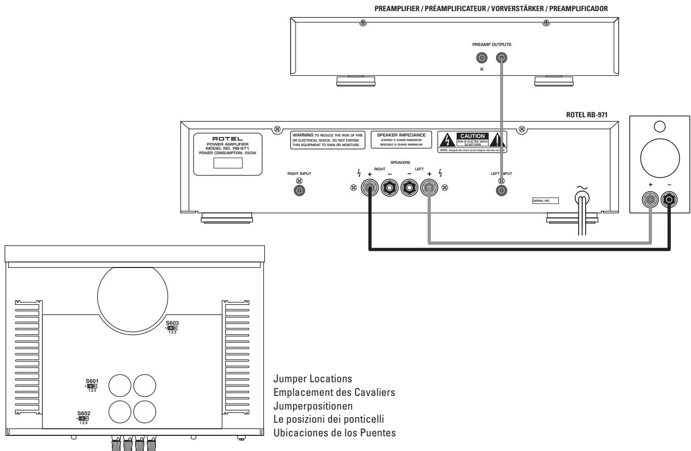
Figure 3: Bridged Mono Connections – Inputs and Speakers Branchements des entrées et des enceintes en ponté mode mono Anschlußdiagramm bei Brückenschaltung - Eingänge und Lautsprecher Collegamenti mono configurazione "a ponte" - Ingressi e diffusori Conexiones para el Funcionamiento en Modo Monofónico Puenteado - Terminales de Entrada y de Conexión a las Cajas Acústicas
