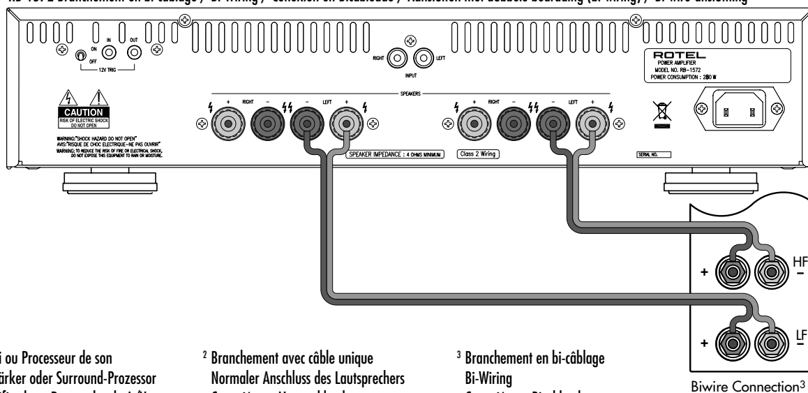
RB-1572 Branchement en bi-câblage / Bi-Wiring / Conexión en Bicableado / Aansluiten met dubbele bedrading (bi-wiring) / Bi-wire-anslutning
