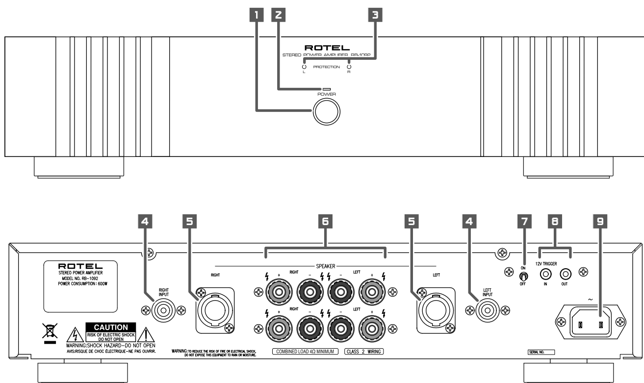
Figure 1: Controls and Connections Commandes et branchements Bedienelemente und Anschlüsse Pannello frontale e posteriore Controles y Conexiones De bedieningsorganen en aansluitingen Kontroller och anslutningar Органы управления и разъемы для подсоединения
