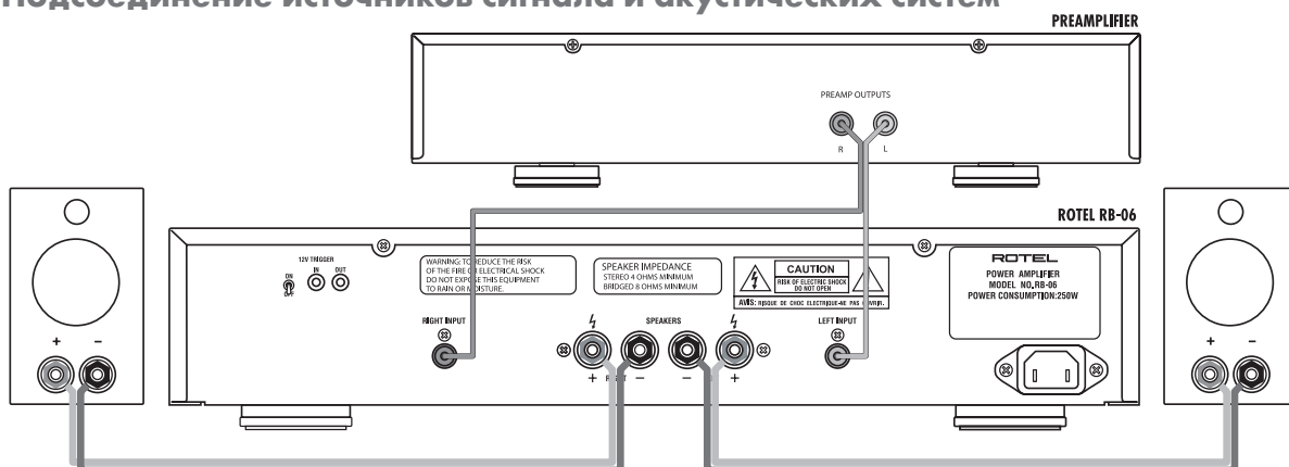
Figure 2: Stereo Connections Branchements stéréo Anschlussdiagramm bei Stereobetrieb Schema dei collegamenti stereo Conexiones de Entrada y de Salida para Funcionamiento en Modo Estereofónico De in- en uitgangsaansluitingen Stereoanslutningar Подсоединение источников сигнала и акустических систем
