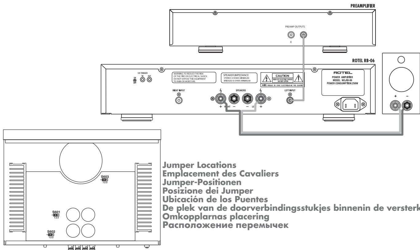
Figure 3: Bridged Mono Connections – Inputs and Speakers Branchements en monophonie – Entrée et enceinte Anschlussdiagramm bei Brückenschaltung – Eingänge und Lautsprecher Schema dei collegamenti mono a ponte – Ingressi e diffusori Conexiones de Entrada y de Salida para Funcionamiento en Modo Monofónico Puenteado De versterker mono schakelen – ingangen en uitgangen Anslutningar – bryggkopplat läge Мостовое включение в режиме моно – подключение входного сигнала и колонок
