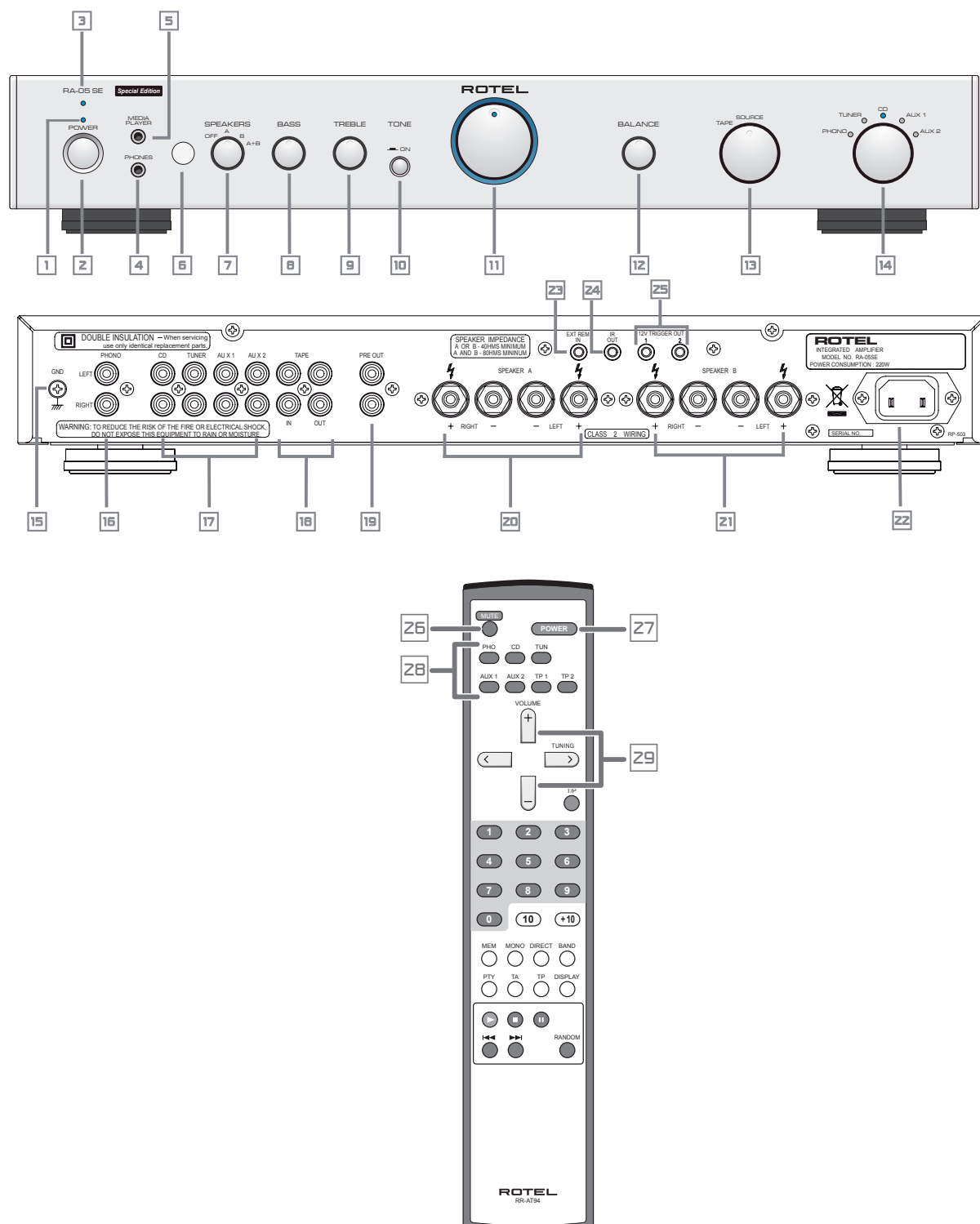
Figure 1: Controls and Connections Commandes et branchements Bedienelemente und Anschlüsse Controles y Conexiones De bedieningsorganen en aansluitingen Controlli e collegamenti Kontroller och anslutningar Органы управления и разъемы
