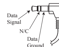
Figure 07– Data Port mini plug
