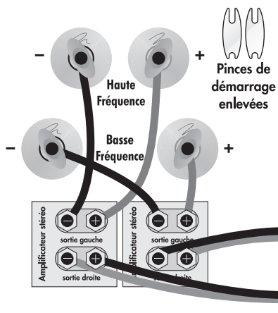
Fig. 3: Raccordement par bi-amplification horizontale. Un canal illustré.
