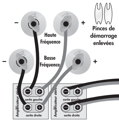
Fig. 4: Raccordement par bi-amplification verticale. Un canal illustré.
