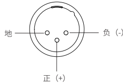
设置反向端口极性示意
