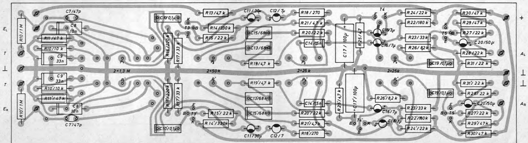
Fig. 11 Ätzschaltplatte 212 606 des Regelverstärkers
