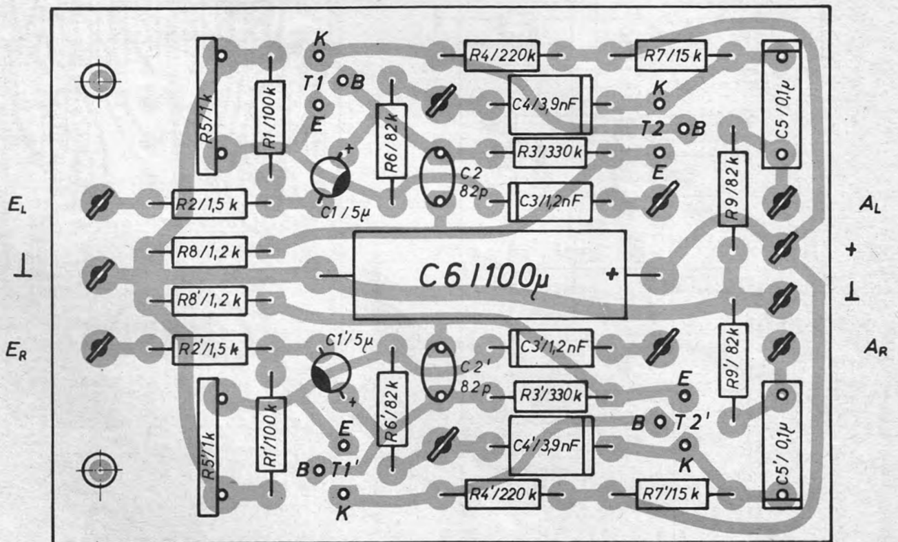
Fig. 8 Ätzschriftplatte 212 605 des Vorverstärkers
