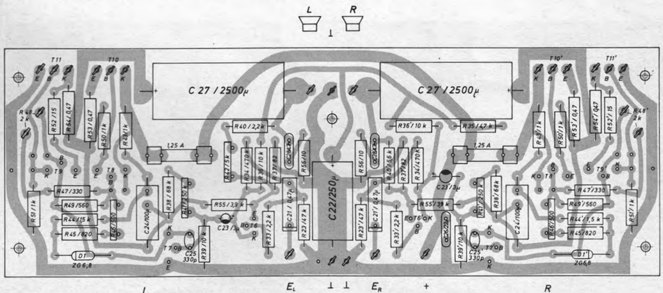
Fig. 13 Ätzsaltplatte 212 603 des Hauptverstärkers (Endstufe)
