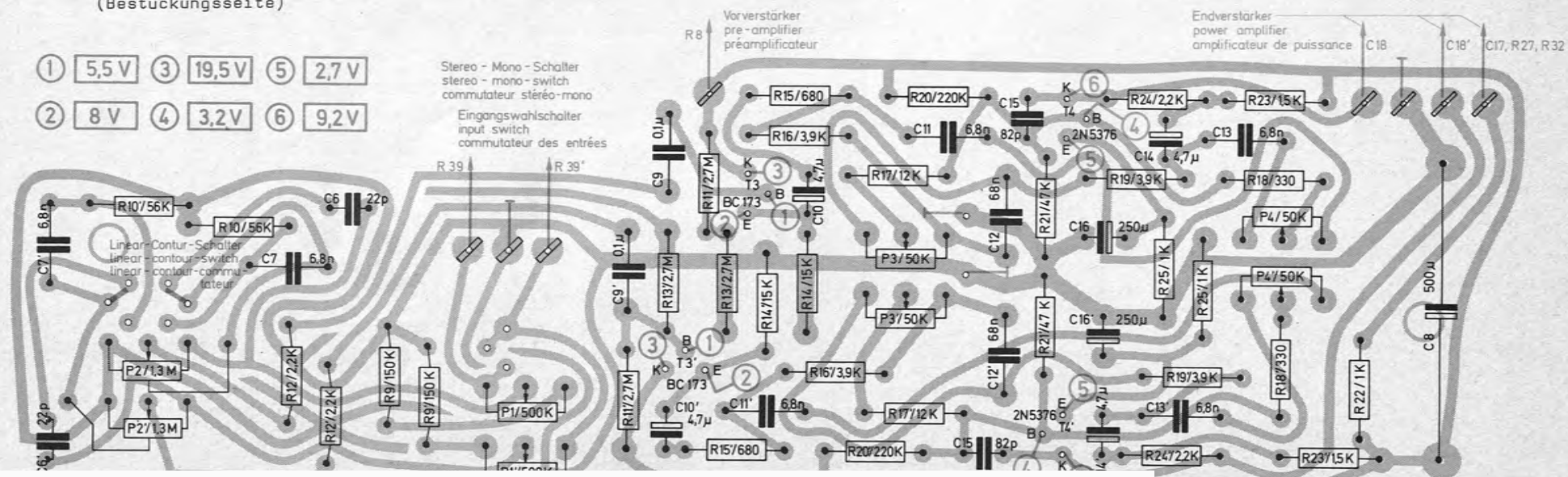
Fig. 9 Ätzsaltplatte des Regelverstärkers 220 225 (Bestückungsseite)
