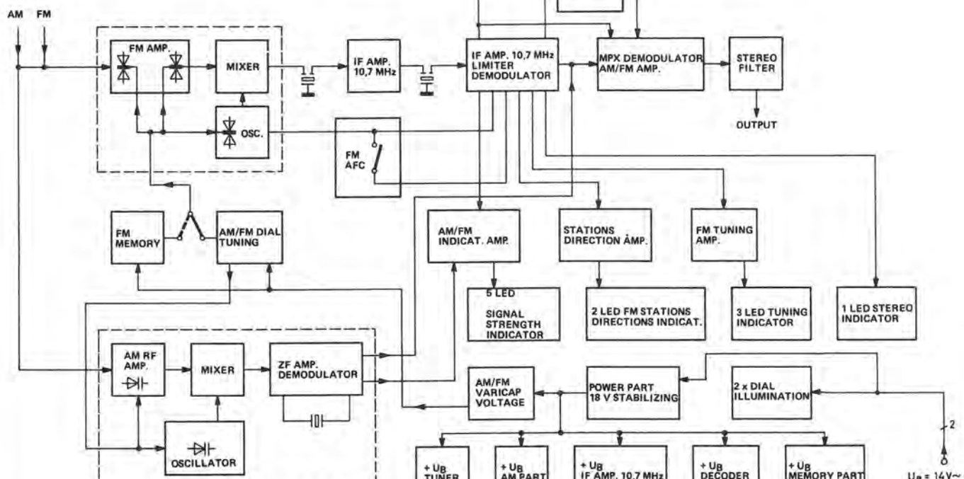
Blockschaltbild CV 1160 Blockdiagram CV 1160 Schéma de bloc CV 1160
