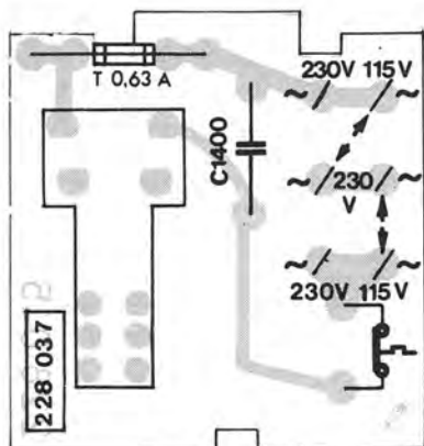
Netzplatte Power board Plaque secteur
