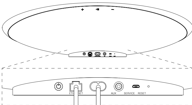
Рисунок 3 Соединение для проводного режима
