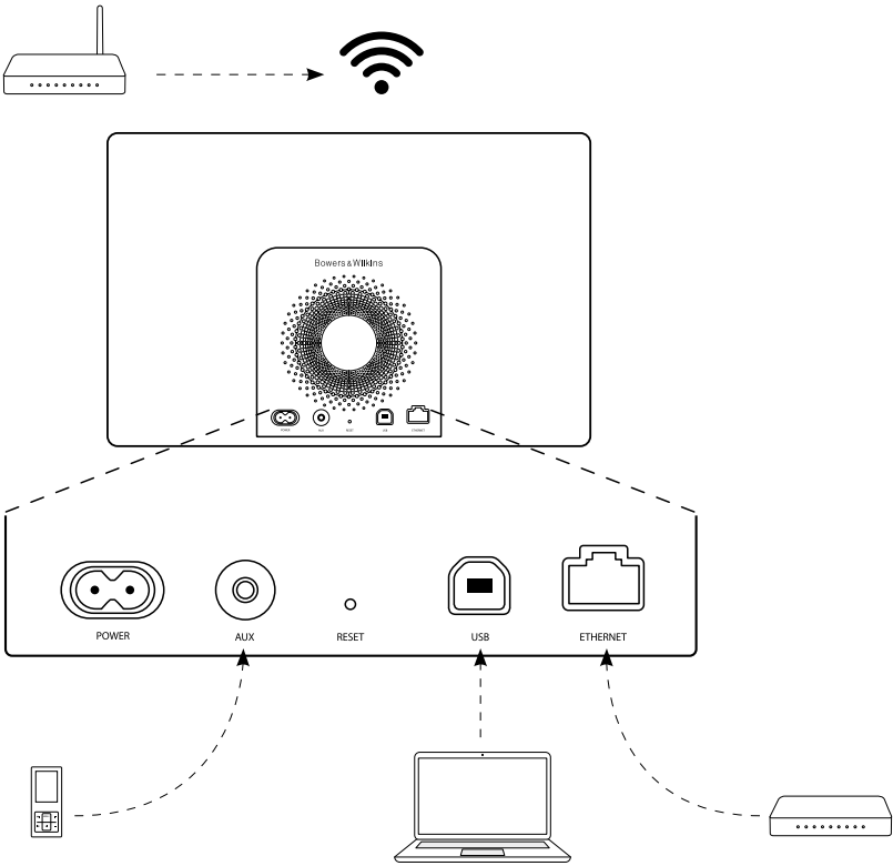
图 5 A7连接
