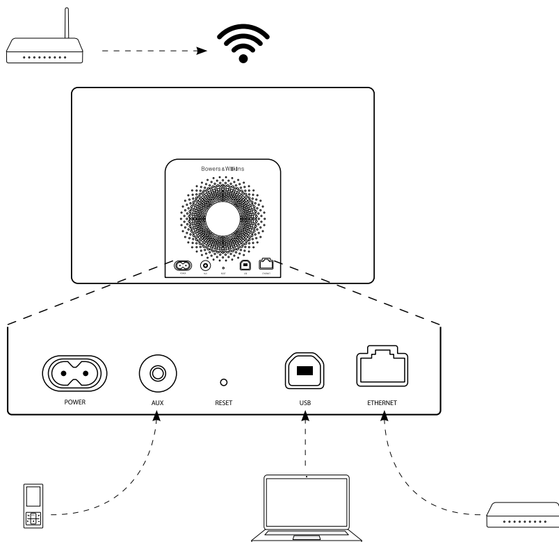
Diagram 5 A7 tilkoblingsmuligheter
