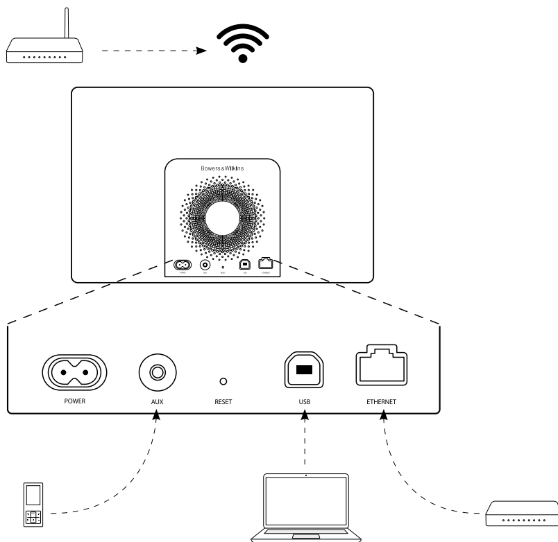
Figura 5 Collegamenti all'A7
