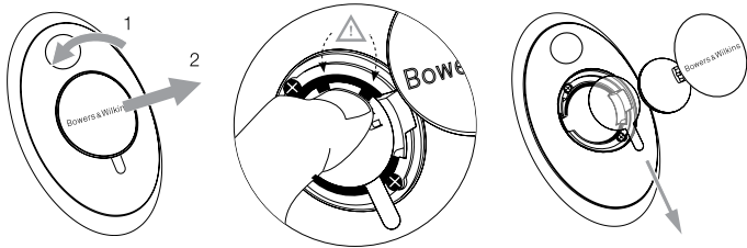
图 3 拆除A7绝缘膜
