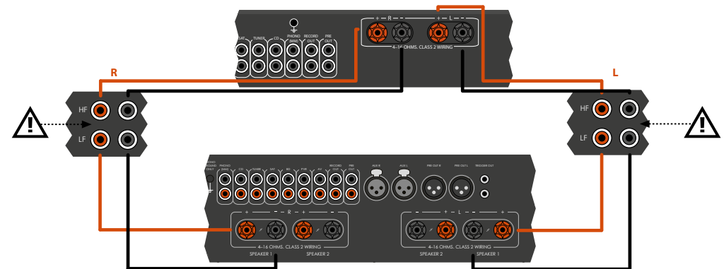
Een A29 en P49 aangesloten op luidsprekers met behulp van bi-amping
